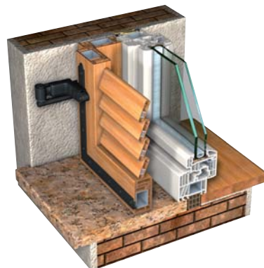
Klappladen mit Rahmenmontage auf Fensterrahmen
