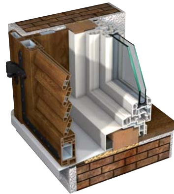
Renovierungsfenster und Klappladen mit Laibungsrahmen
