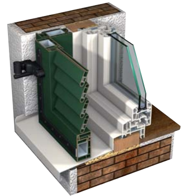
Renovierungsfenster und Klappladen mit Rahmenmontage auf bestehenden Fensterrahmen
